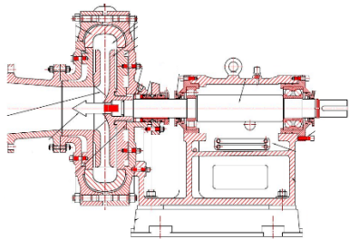
Bombas Para Lodos MP Horizontales
